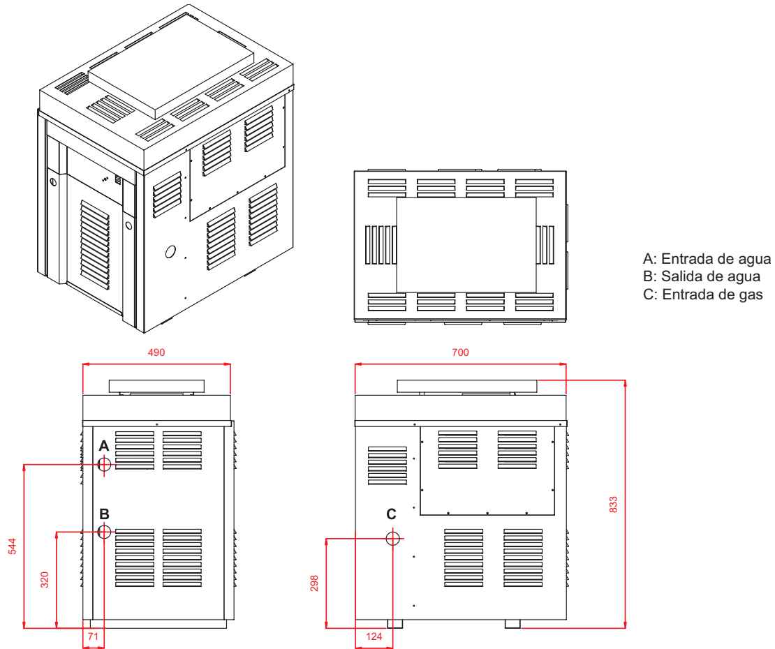
Fig. 1 TX70
