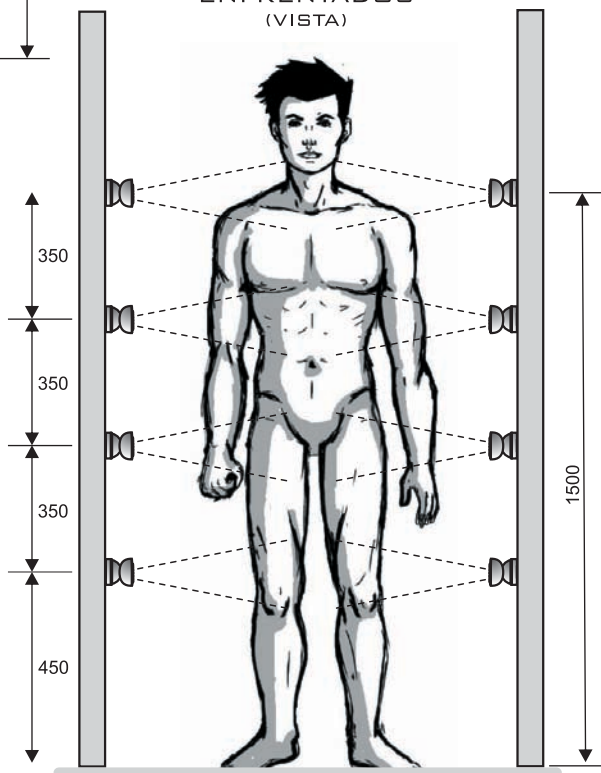
ENFRENTADOS (VISTA)
